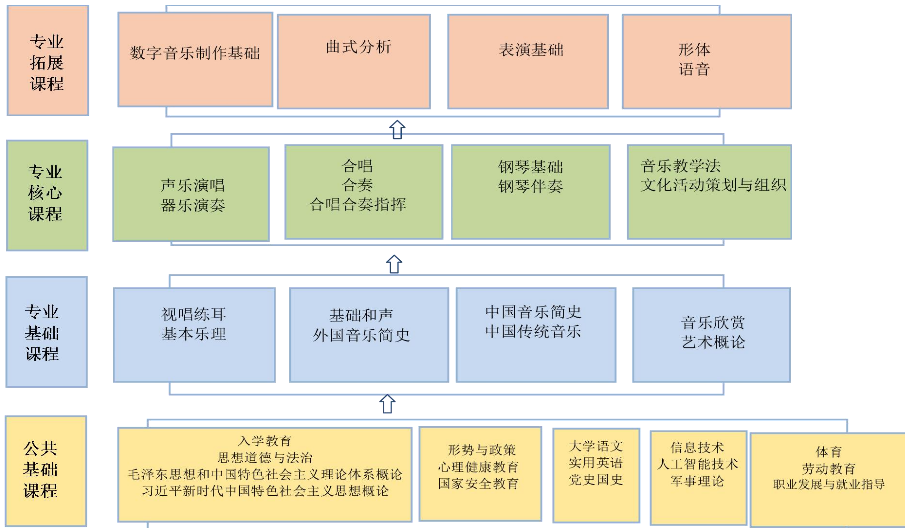
图 1 课程结构图
